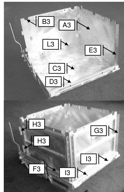
Abbildung 4.3 – Montage Seitenteile
