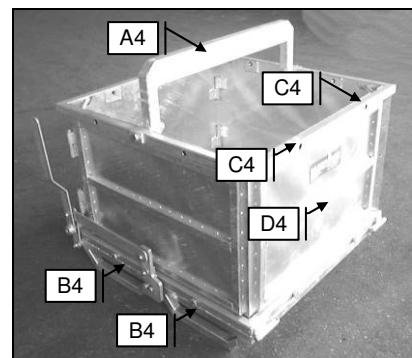
Abbildung 4.4 – Montage Rahmen
