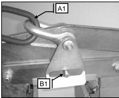
Abbildung 5.1 – Plattengreifer R 1500 gesichert und einsatzbereit
