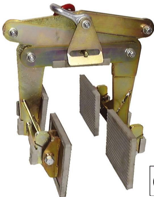
Abbildung 1 Gesamtansicht Plattengreifer R 1500
