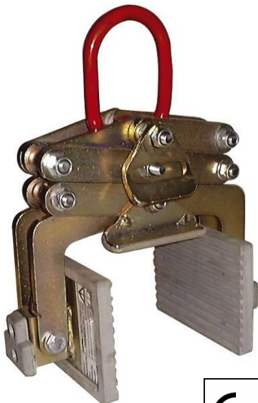
Abbildung 1 Gesamtansicht Plattengreifer R 400
