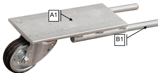
Abbildung 5.1 Montage des Verlängerungssatzes
