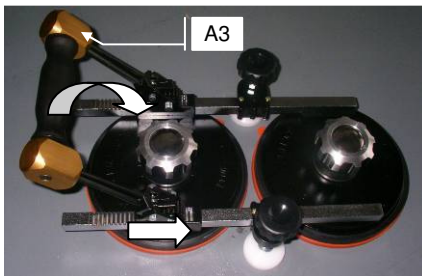
Abbildung 5.3 – Verschieben mit dem Saugheber Mammut
