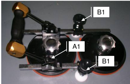
Abbildung 6.1 – Saugheber Mammut
