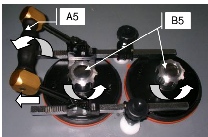
Abbildung 5.5 – Lösen des Saughebers Mammut
