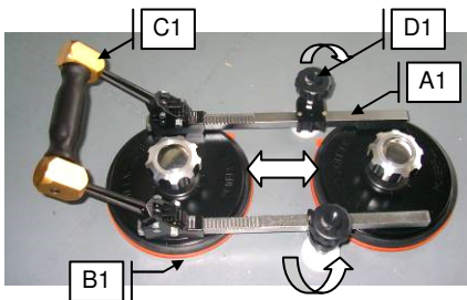
Abbildung 5.1 – Aufsetzen des Saughebers Mammut
